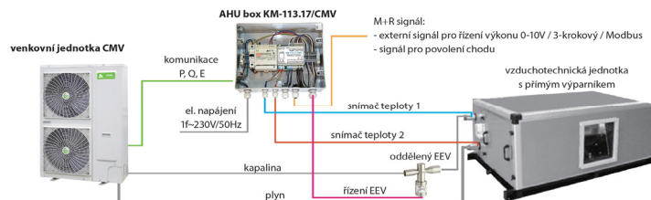
Schéma přepojení CMV:
