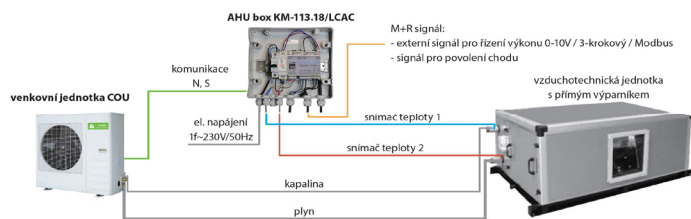
Schéma přepojení LCAC:
